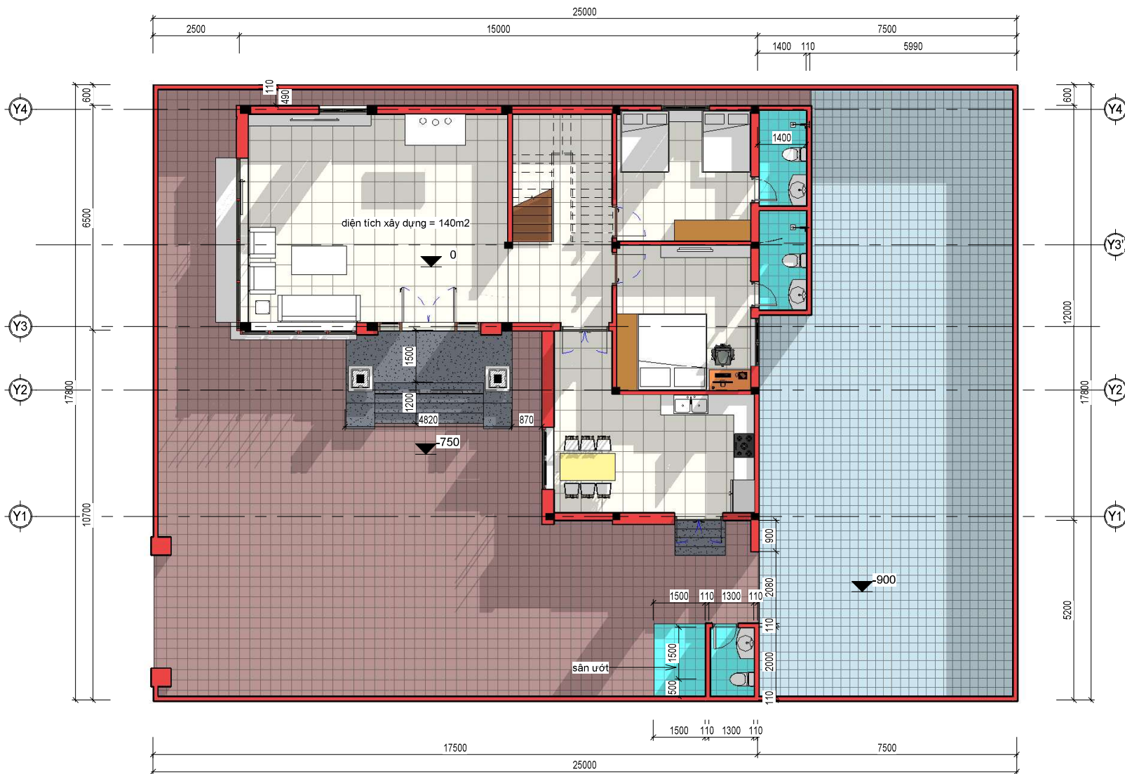
1 MẶT BẰNG TỔNG THỂ 1 : 100
