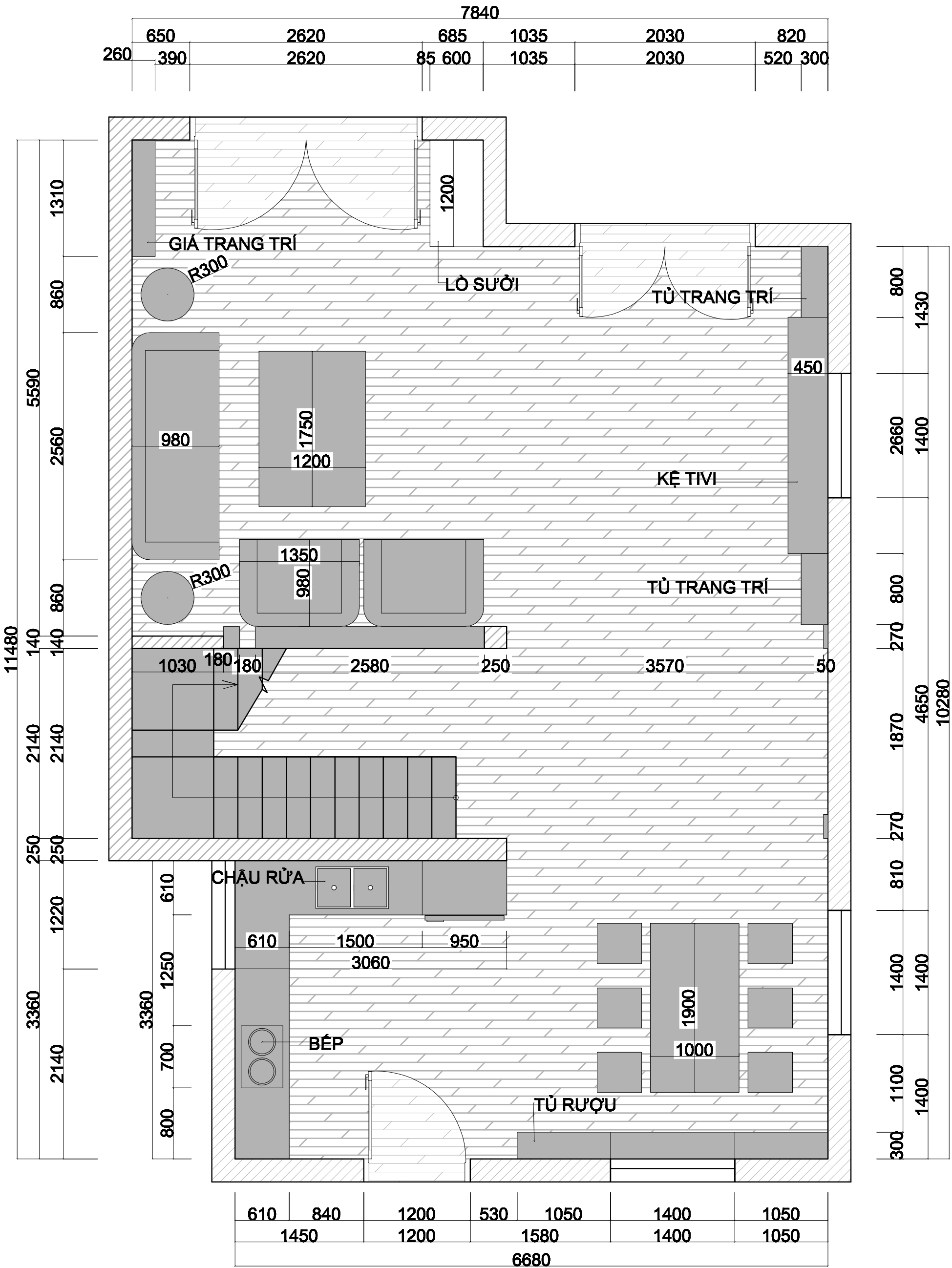
MẶT BẰNG BỐ TRÍ NỘI THẤT TẦNG 1
