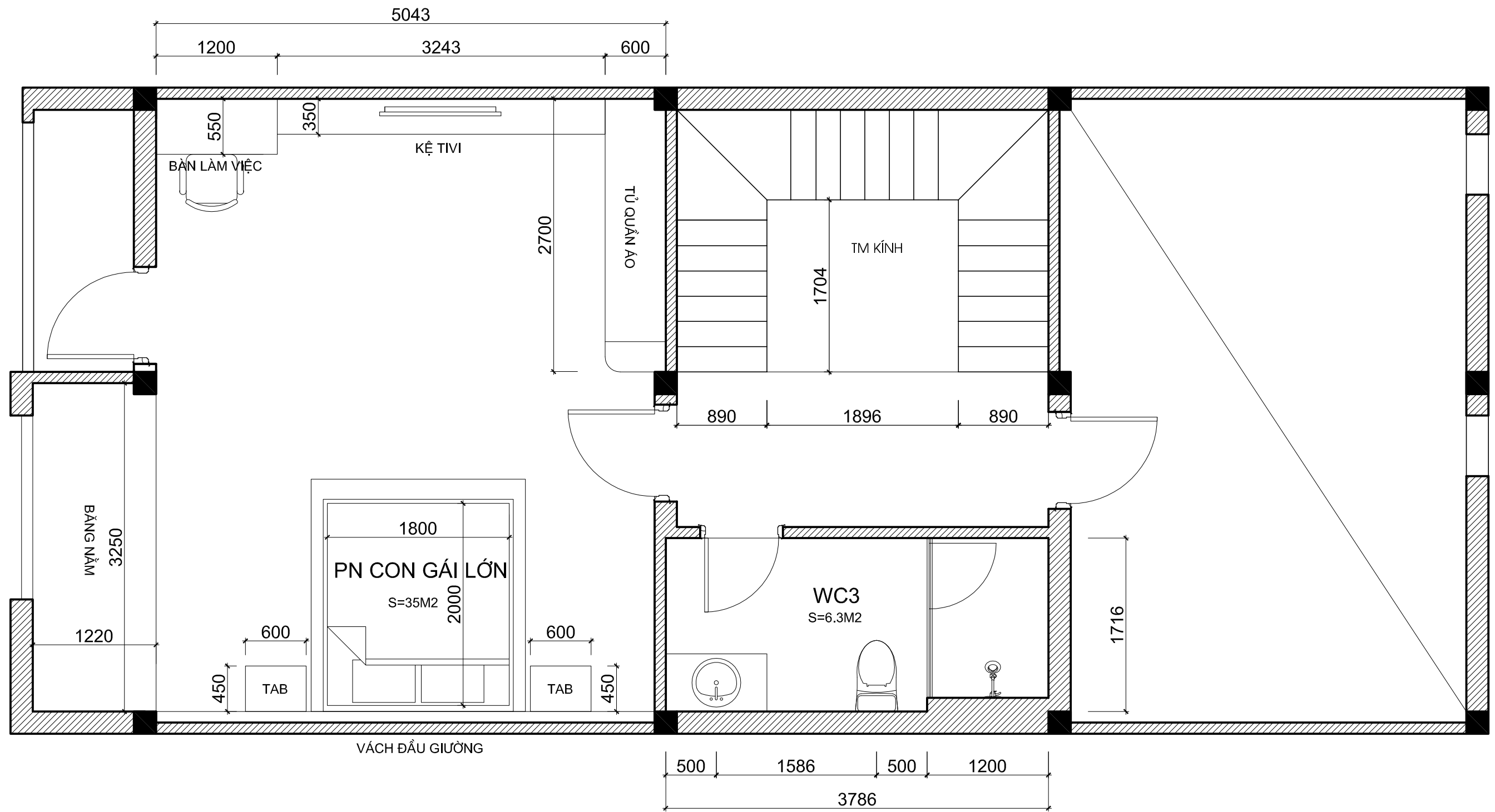
MẶT BẰNG TẦNG 3
