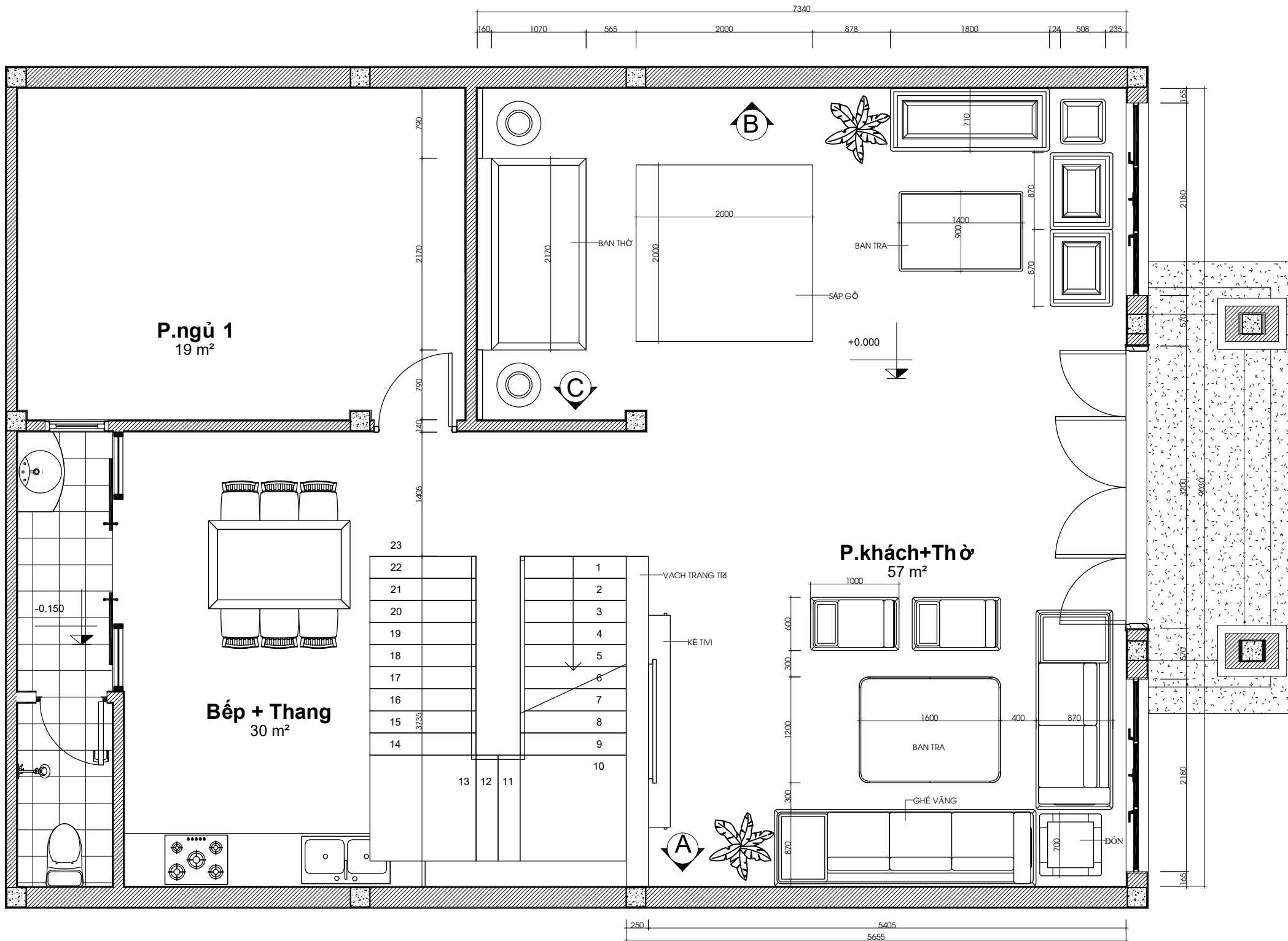
MẶT BẰNG NỘI THẤT P KHÁCH + THỜ
