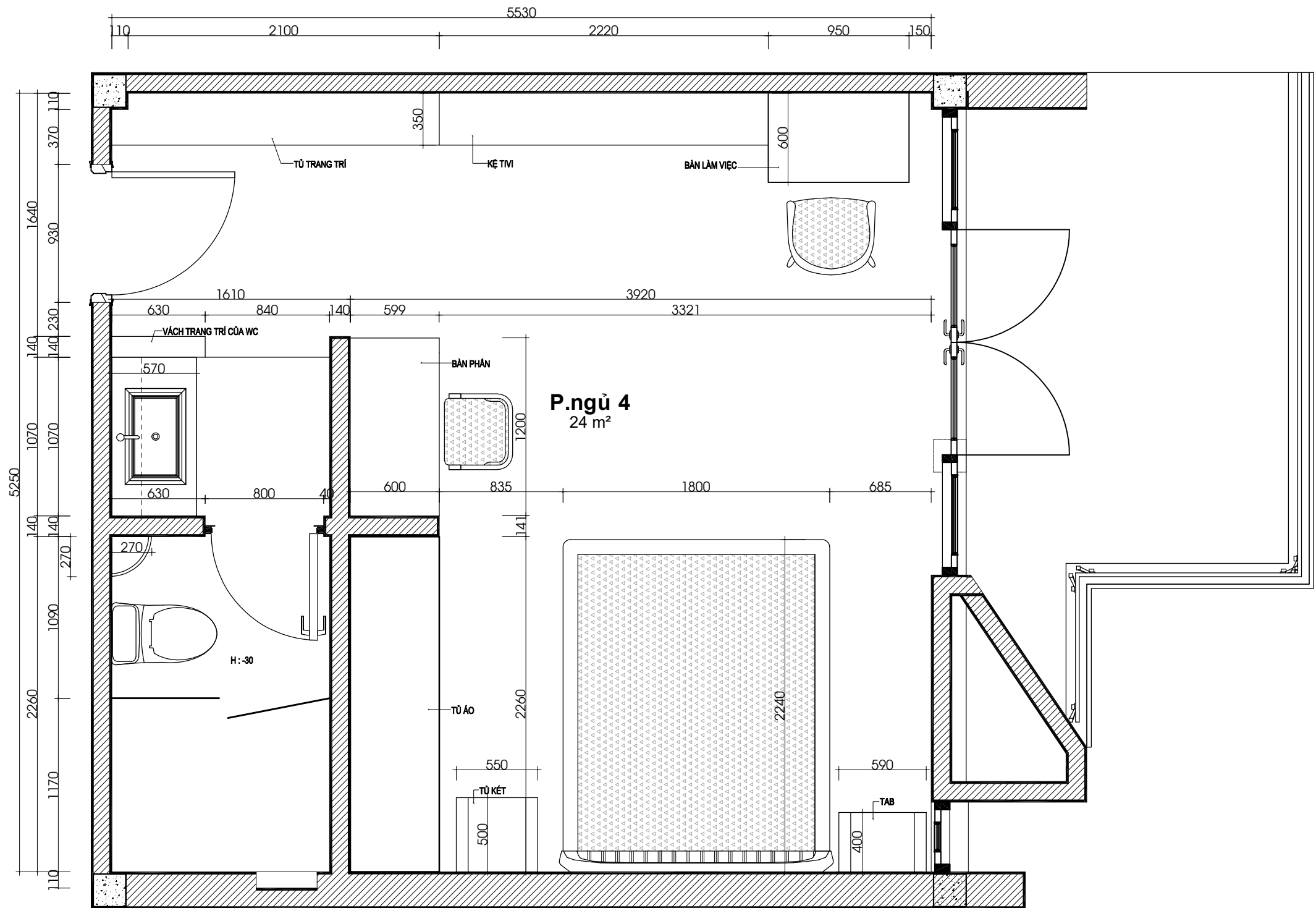
MẶT BẰNG BỐ TRÍ NỘI THẤT PHÒNG NGỦ
