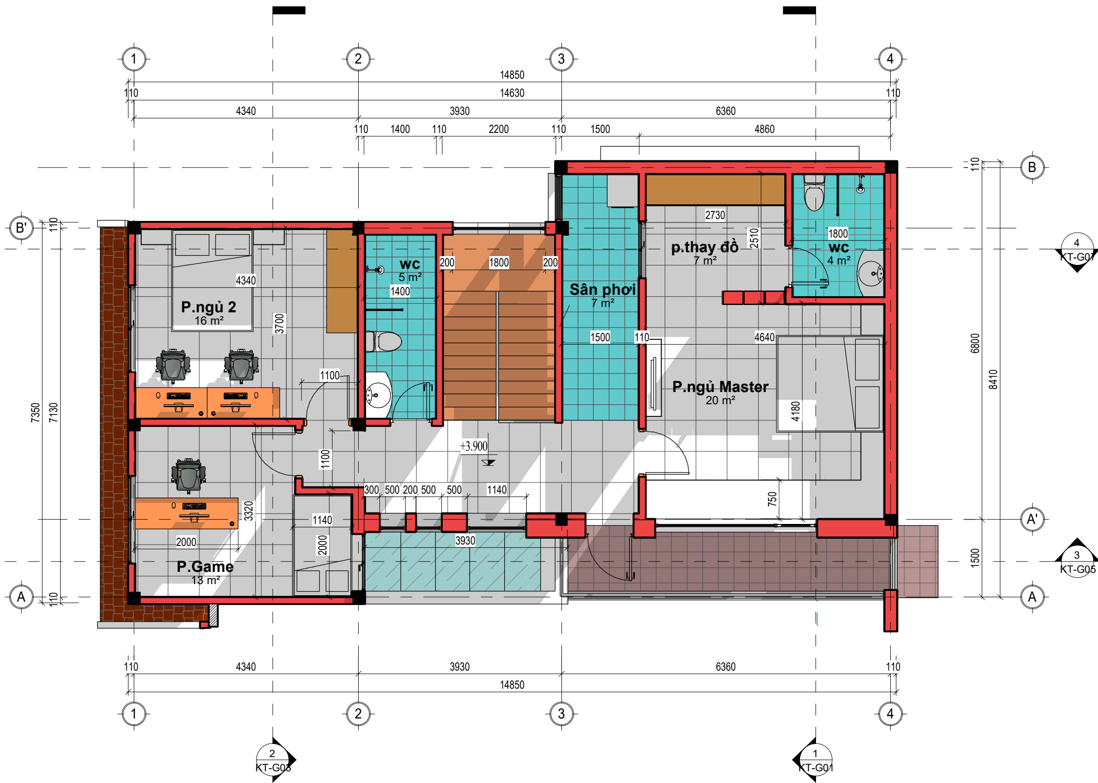
1 MẶT BẰNG NỘI THẤT TẦNG 2 1:70
