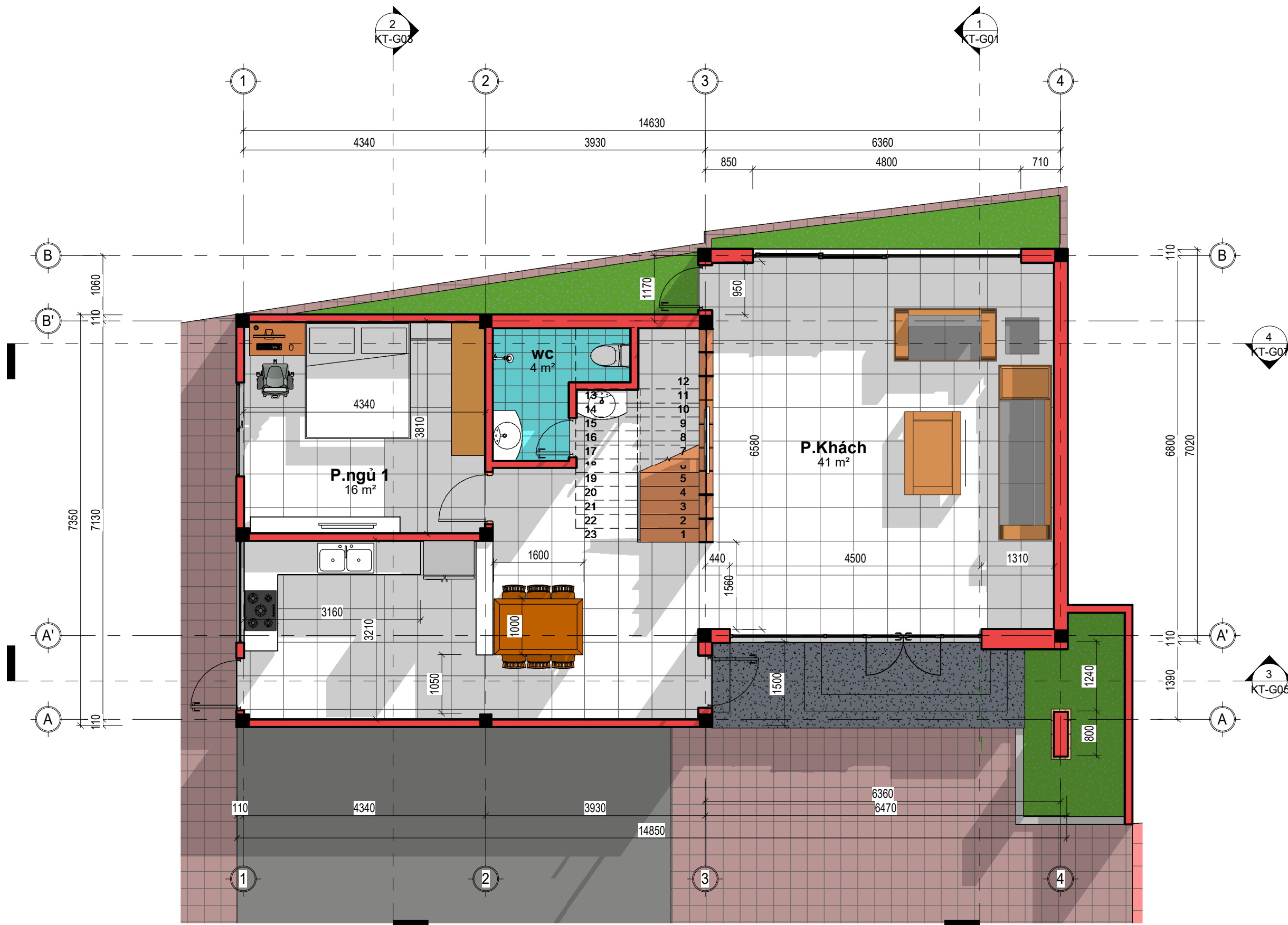
1 MẶT BẰNG NỘI THẤT TẦNG 1 1 : 70
